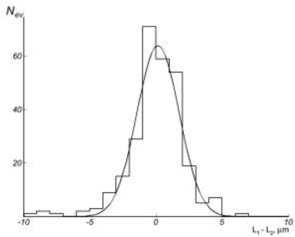
Рис. 10. Распределение пробегов L_1 и L_2 в парах \alpha -частиц.
