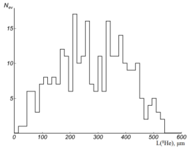
Рис. 7. Распределение следов ^8\text{He} по длине пробега в эмульсии.
