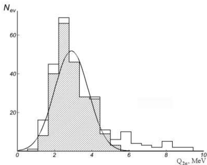
Рис. 11. Распределение разностей пробегов в парах \alpha -частиц L_1 - L_2 ; линия – функция Гаусса.
