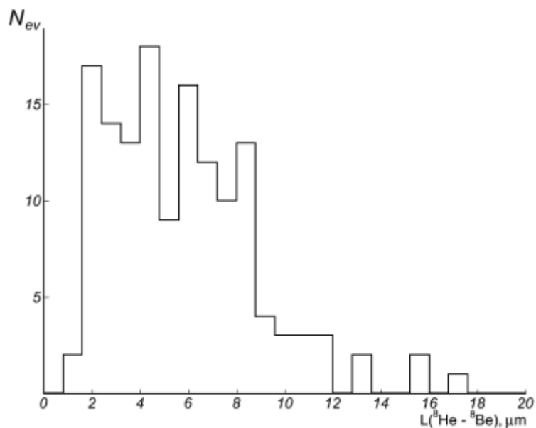
Рис. 13. Распределение по расстояниям L(^8\text{He} - ^8\text{Be}) между точками останова ядер ^8\text{He} и вершинами распадов ^8\text{Be} (2^+) в «разорванных» событиях.
